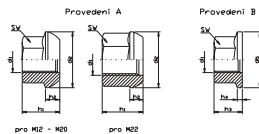
Maticе kolové provedení A a B
